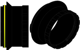
Art. Nr. UWFP DISTANZD138L020 Bez1. Distanzring für 138 Flansch auf 129 Port Bez2. von Bajonett 138 auf Bajonett 129
