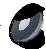
Art. Nr. UWFP DOME D215 PL Bez1. Domeport 8,03 Zoll Kugeldurchmesser aussen Plexigl Bez2. Abschnitt 215, Vollformat Fisheye
