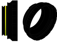
Art. Nr. UWFP DISTANZD106L020 Bez1. Distanzring für 106 Flansch auf 129 Port Bez2. von Bajonett 106 auf Bajonett 129
